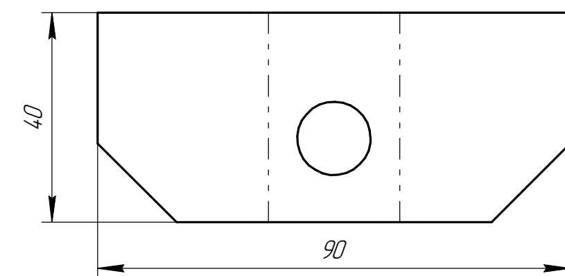
Дет. поз. 6 (1:1)
