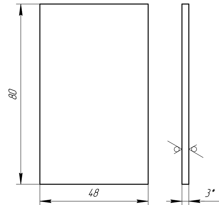
Дет. поз. 2 (1:1)
