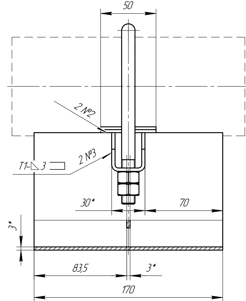
Дет. поз. 2 (1:1)
