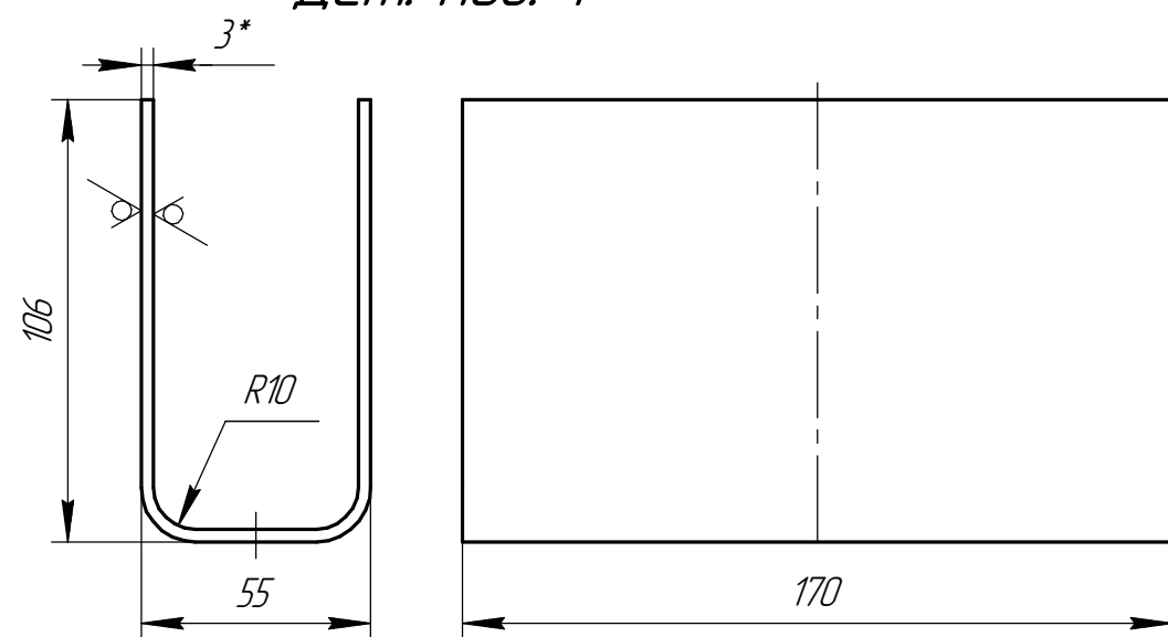
Дет. поз. 1
