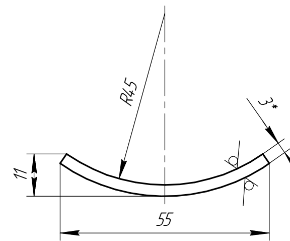
Дет. поз. 4 (1:1)
